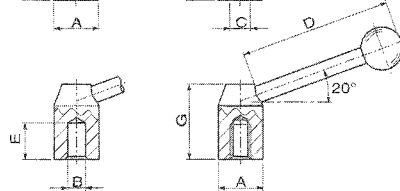
Type B 傾斜把手 Inclined handle
