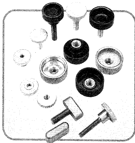
8080 平頭壓花螺帽 Flat Knurled Nuts P.111
