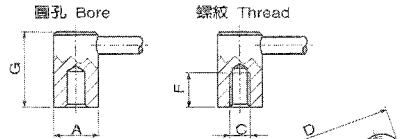
Type A 水平把手 Horizontal handle
