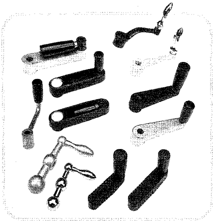
曲柄把手 Cranked Handles P.39
